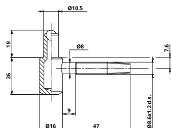
Cilindrična spojnica CG075130H004 / Hinge CG075130H004
