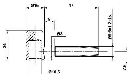
Cilindrična spojnica CF075130H004 / Hinge CF075130H004
