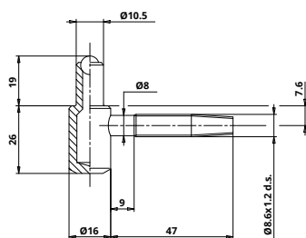
Cilindrična spojnica CG055160H106 / Hinge CG055160H106
